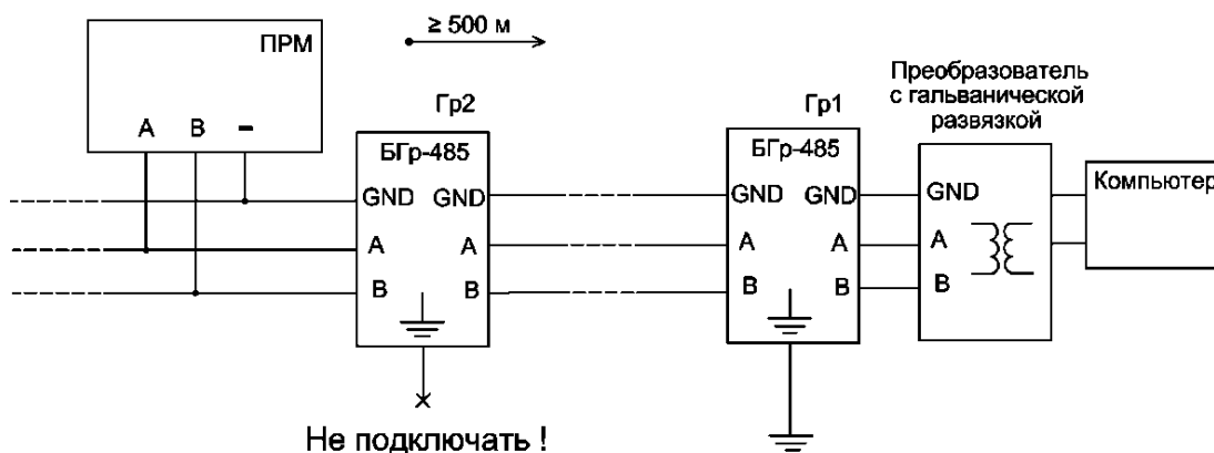
Рисунок 2.12 – Пример обеспечения грозозащиты линии RS-485
